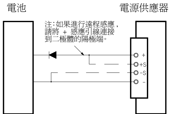
圖 3-1. 電池充電的建議保護電路
