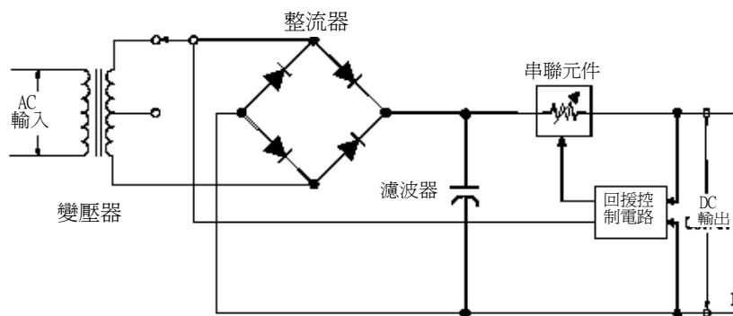
圖 7-1. 含分接調節器的簡式串聯電源供應器線路圖
