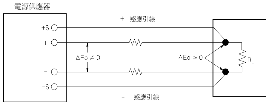
圖 7-7. 具有遠程感應功能的調節式電源供應器
