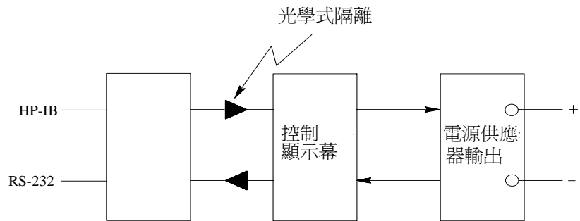
圖 7-2. 電源供應器的方塊圖顯示光學式隔離
