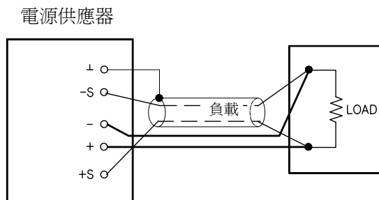
圖 3-2. 遠程電壓感應連接
