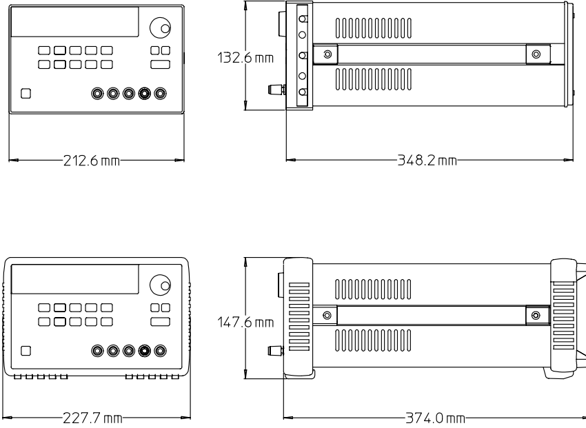
圖 8-1. Agilent E3632A 電源供應器的尺寸
