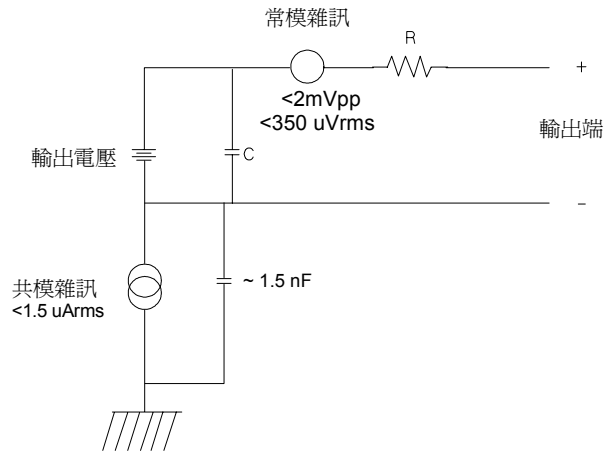
圖 7-6. 共模和常模雜訊源的簡圖
